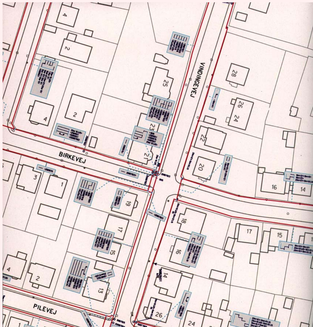
Διάγραμμα Δικτύων Κοινής Ωφέλειας
