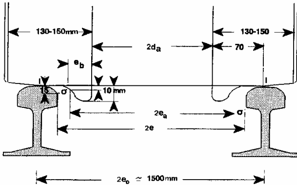
Σιδηροδρομικοί τροχοί επί σιδηροτροχιών. Γεωμετρικά και κατασκευαστικά μεγέθη
