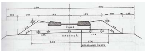
Διατομή μονής γραμμής με διμερείς στρωτήρες - ευθυγραμμία
