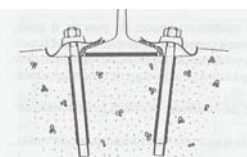
Σχ. 6.18. Ελαστικός σύνδεσμος κοιλωτής μορφής
