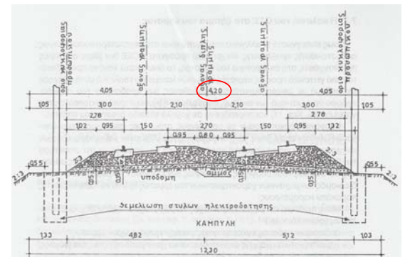
Διατομή διπλής γραμμής με διμερείς στρωτήρες - καμπύλη
