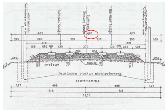
Διατομή διπλής γραμμής με διμερείς στρωτήρες - ευθυγραμμία
