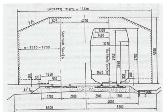
Περιτύπωμα για συρμούς υψηλών ταχυτήτων
