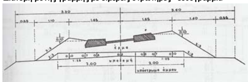
Διατομή μονής γραμμής με διμερείς στρωτήρες - καμπύλη
