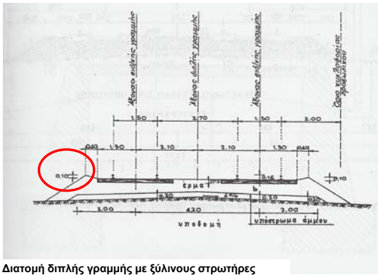
Διατομή διπλής γραμμής με ξύλινους στρωτήρες
