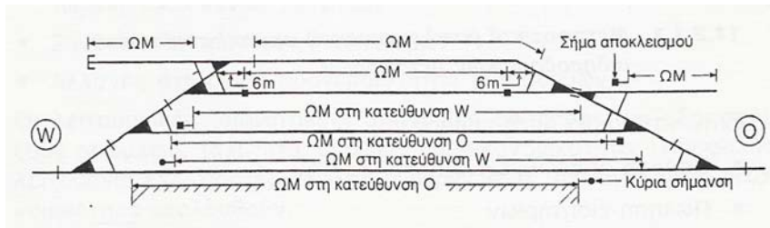
Ωφέλιμο μήκος γραμμών ( \Omega M )
